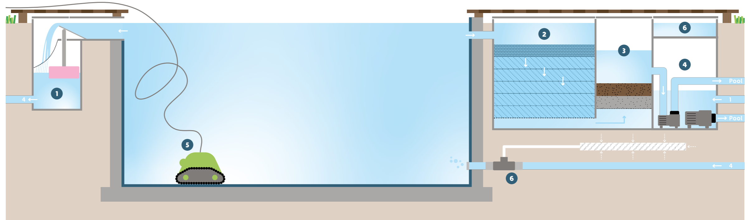
↑ Schematischer Querschnitt
